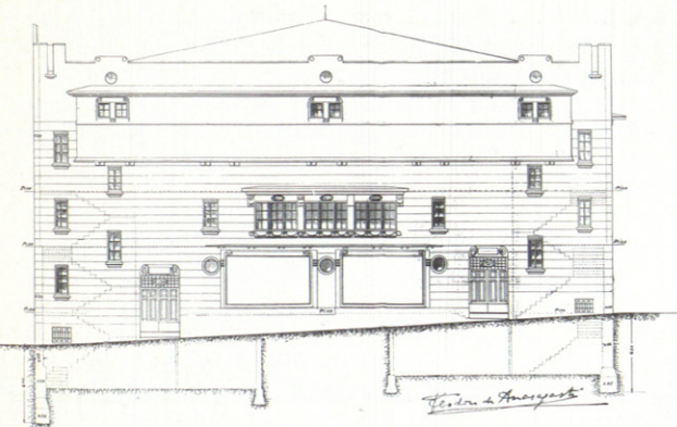
FACHADA POSTERIOR ESCALA DE 1:100
