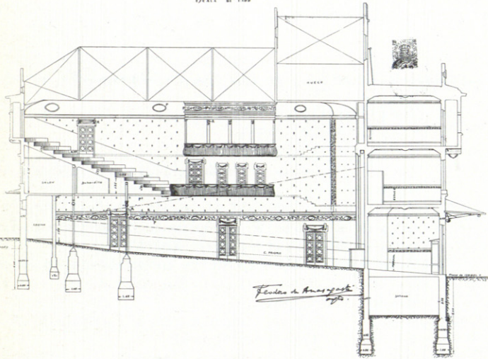
PROYECTO DE CINEMATÓGRAFO PARA LA PLAZA DE ISABEL II - N.º 8 CORTE LONGITUDINAL ESCALA DE 1:100
